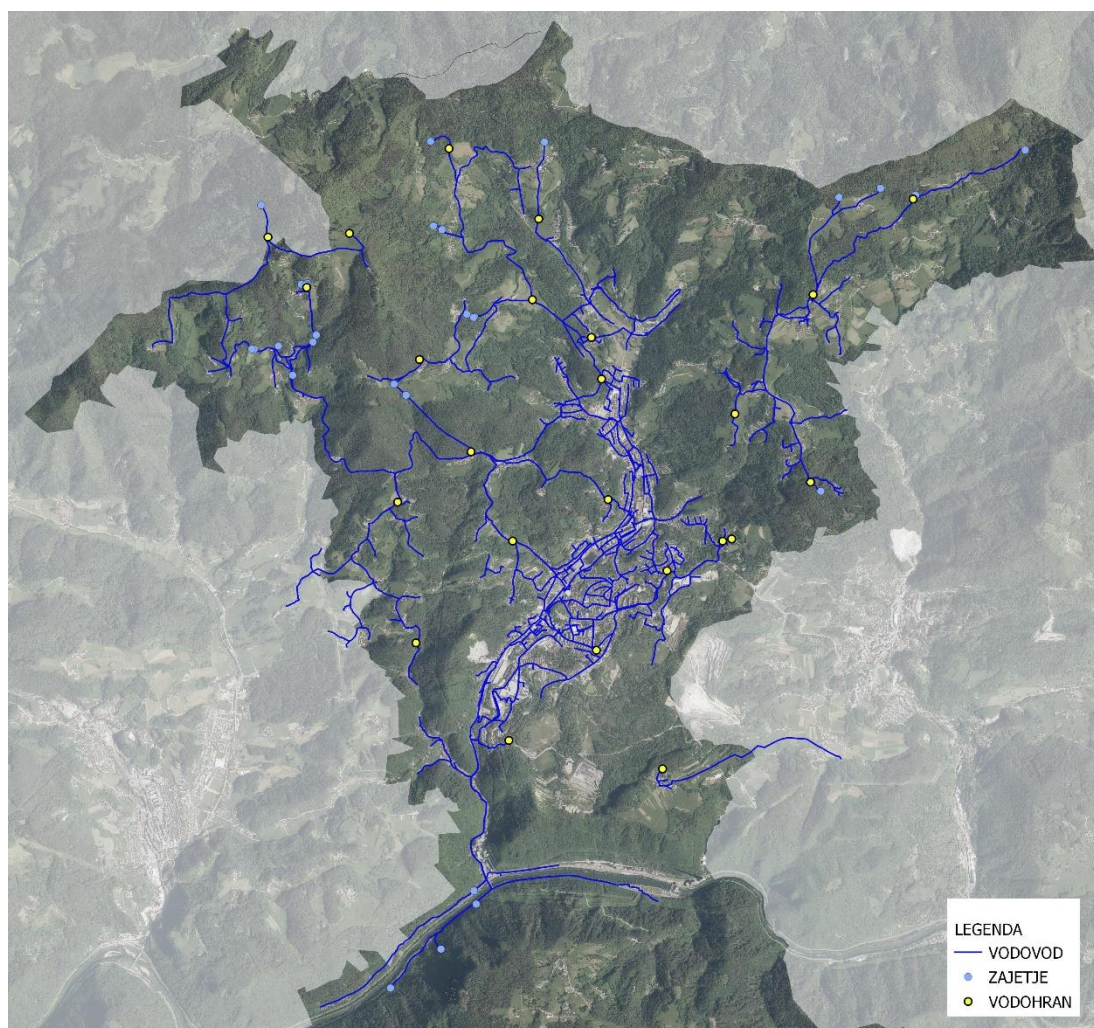
Slika 1: Objekti v sistemu Javnega vodovoda Trbovlje
